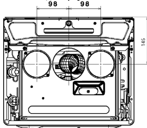
Вид сверху на котел
